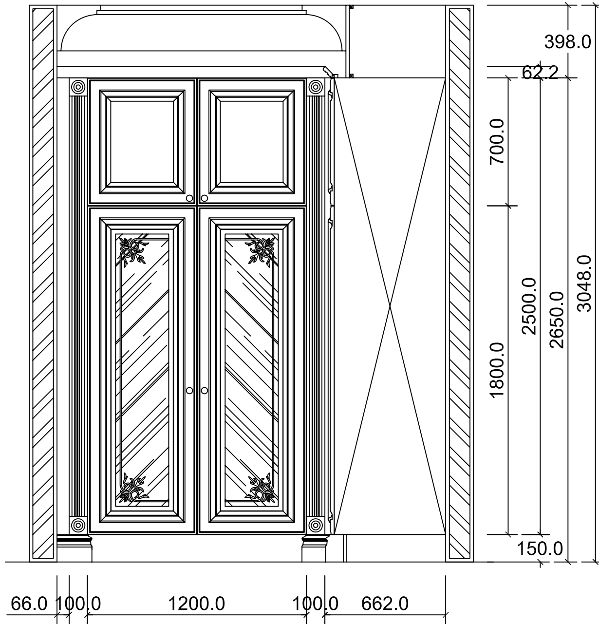
ELEVATION B
