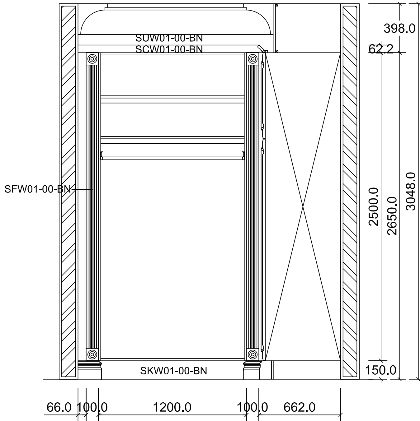
ELEVATION B
