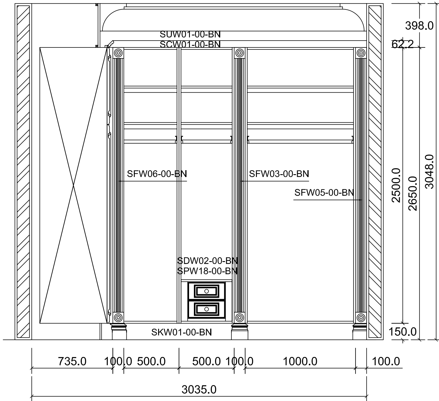
ELEVATION A
