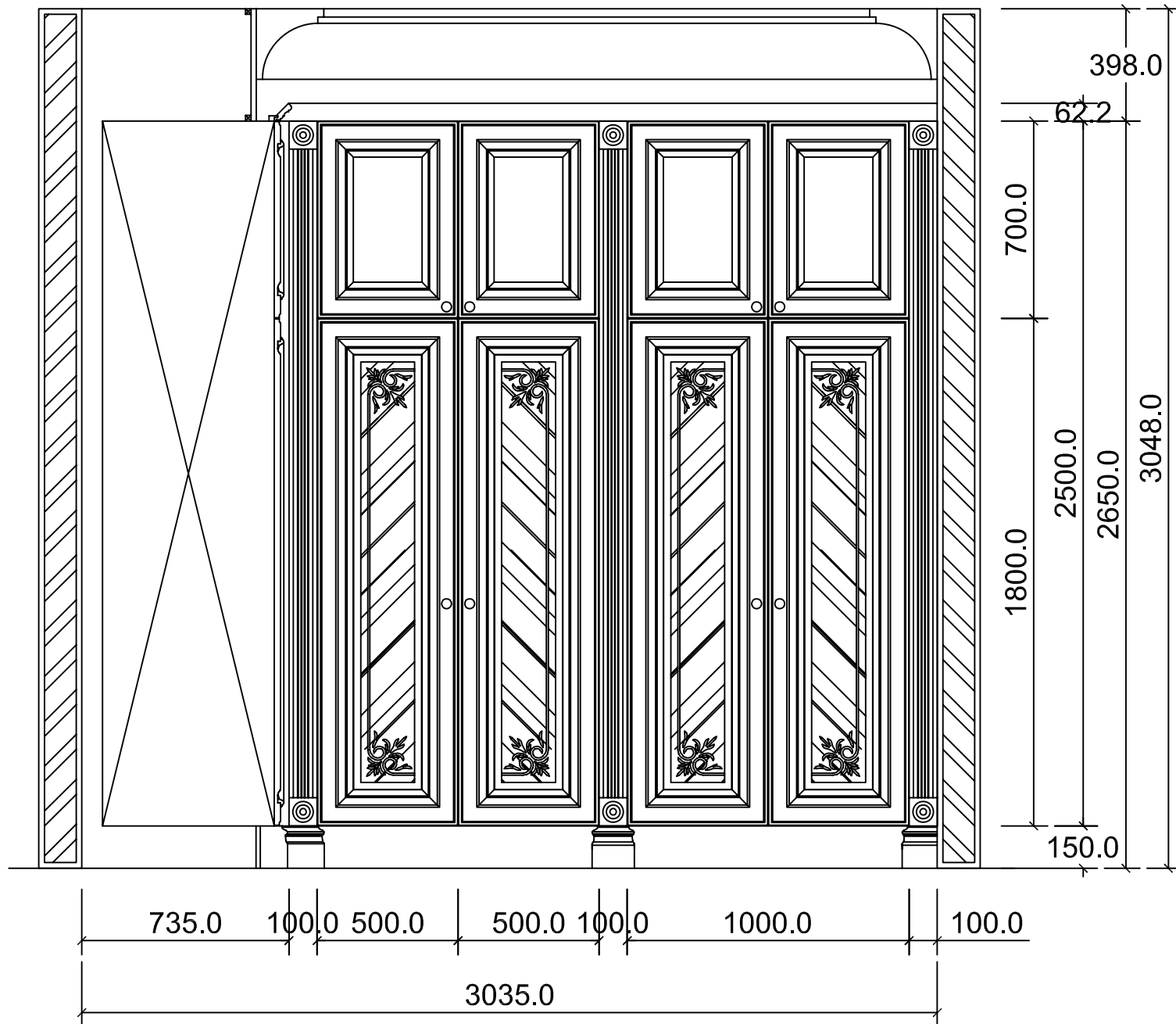
ELEVATION A
