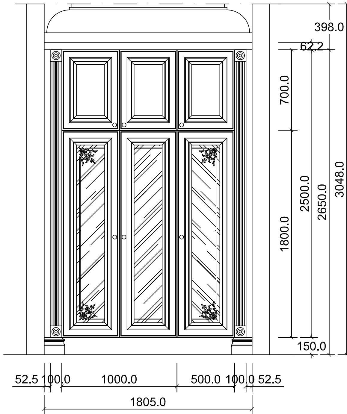
ELEVATION A
