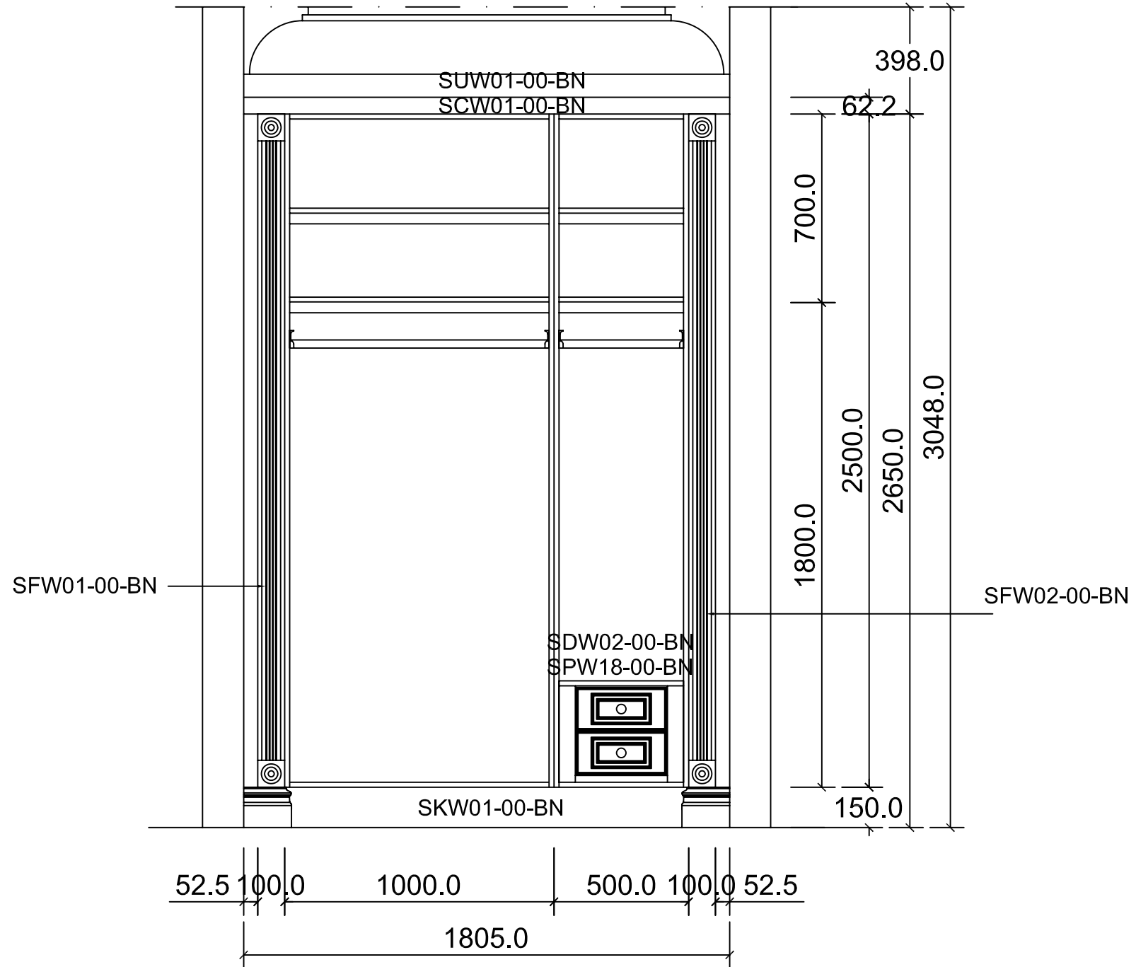
ELEVATION A
