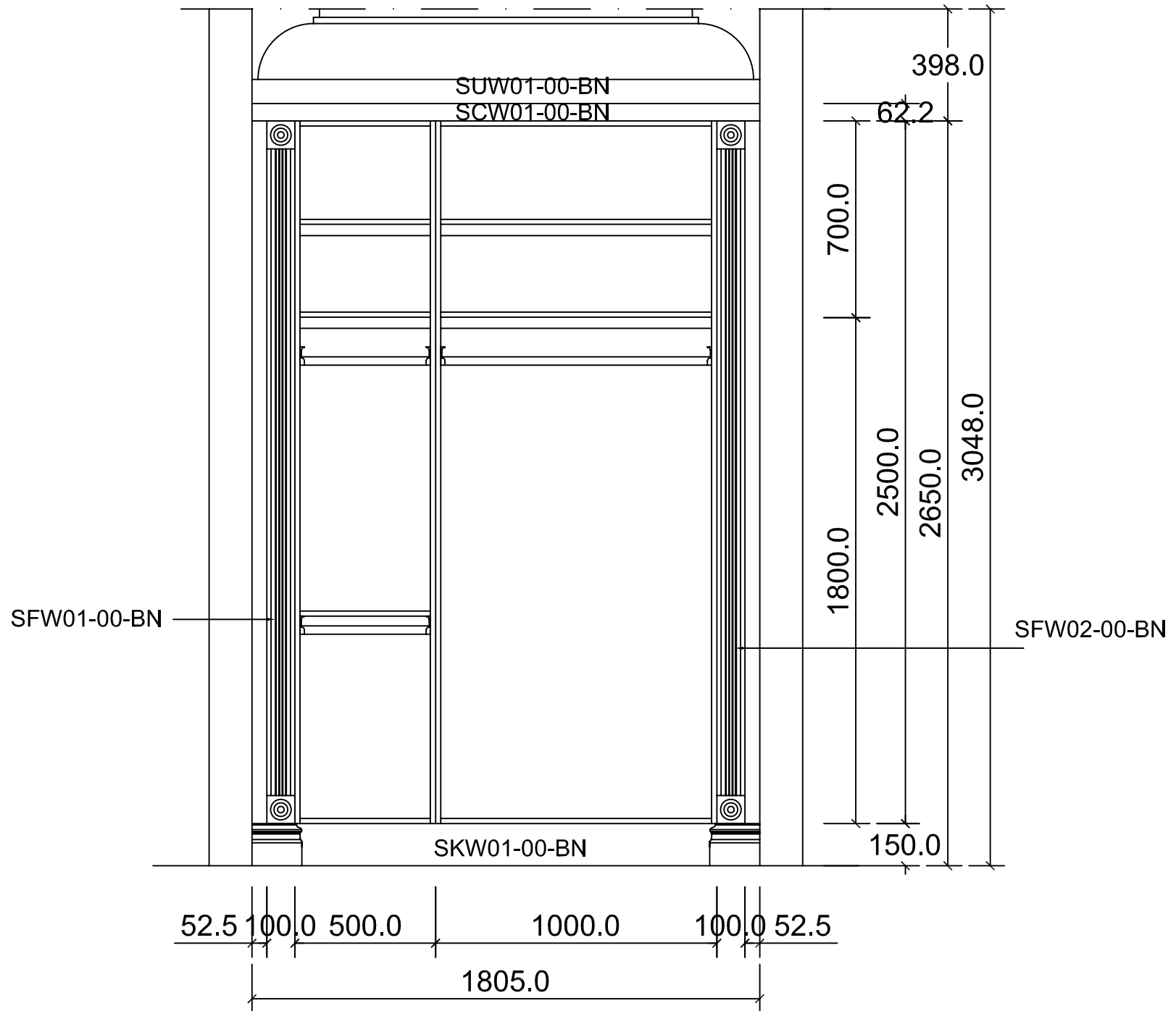
ELEVATION B
