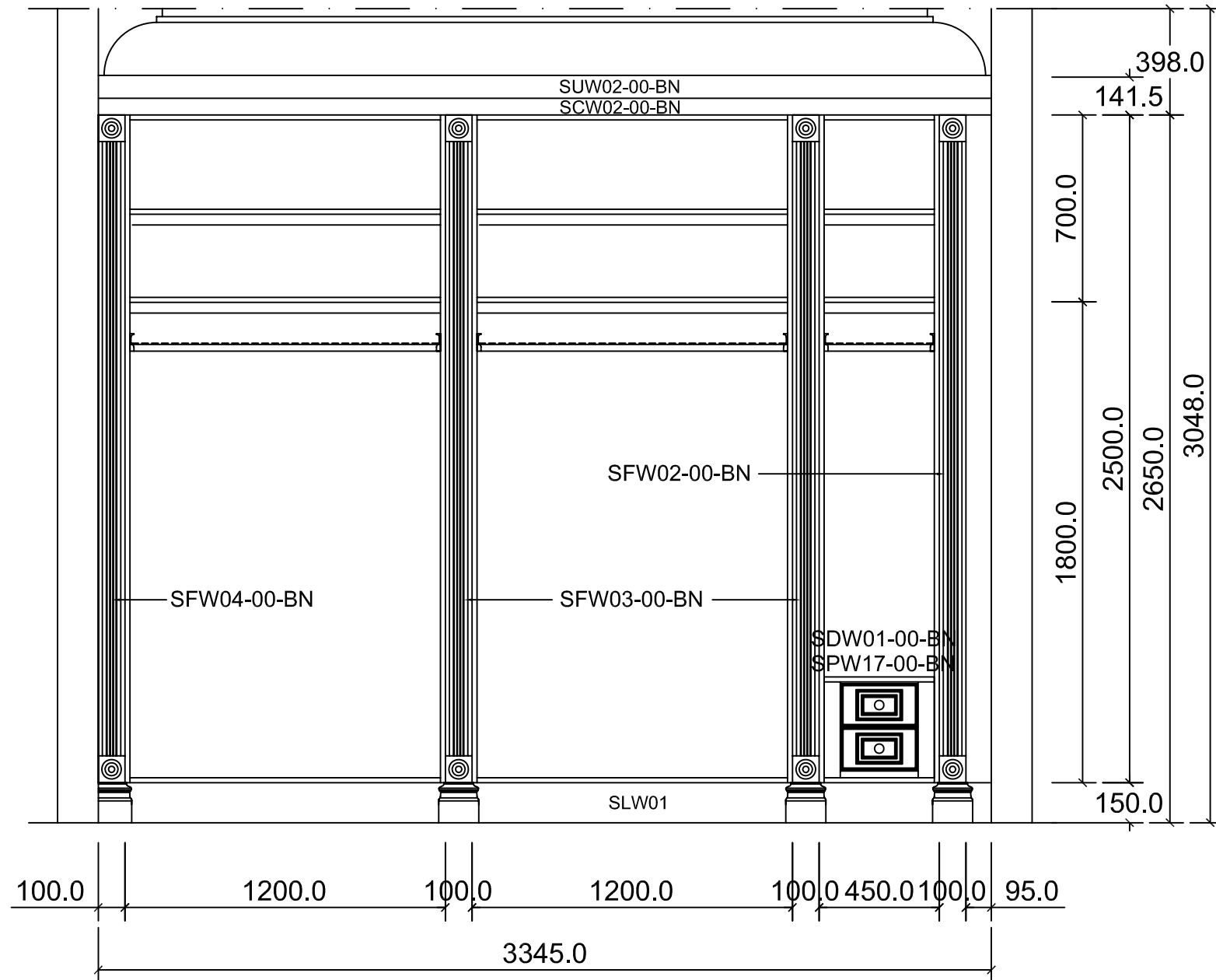
ELEVATION A
