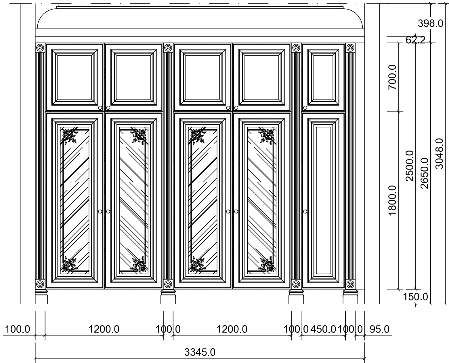
ELEVATION A
