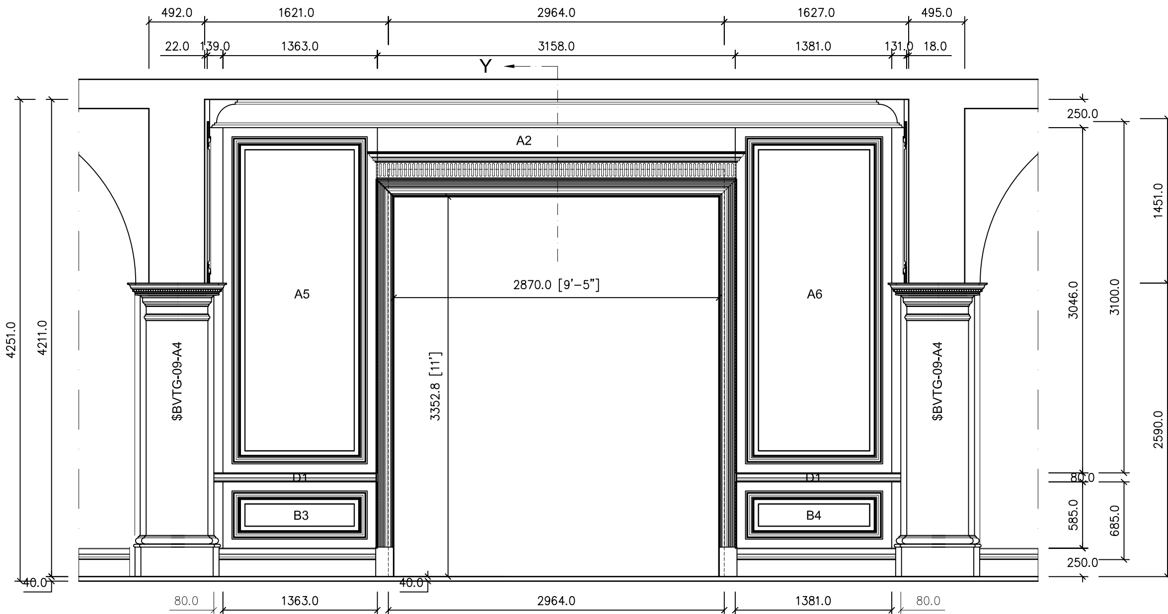
ELEVASI - C Skala 1 : 1
