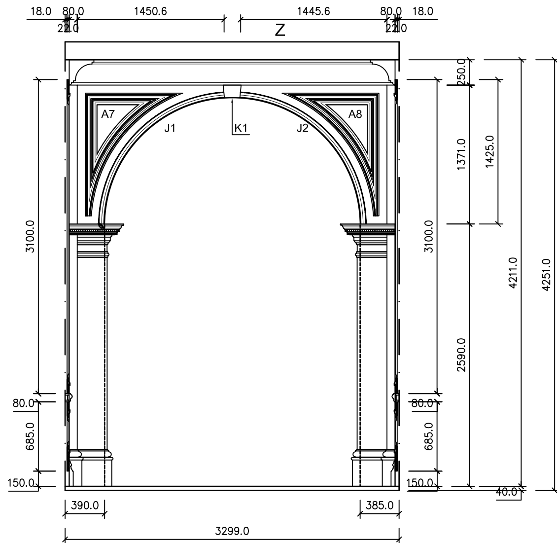
ELEVASI - D Skala 1 : 1
