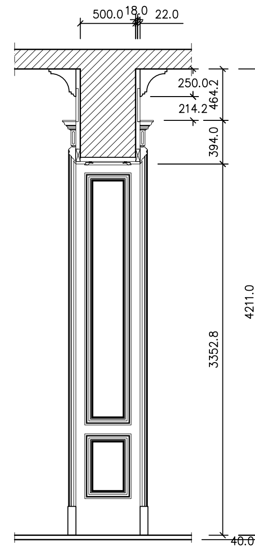
POTONGAN Y Skala 1 : 1
