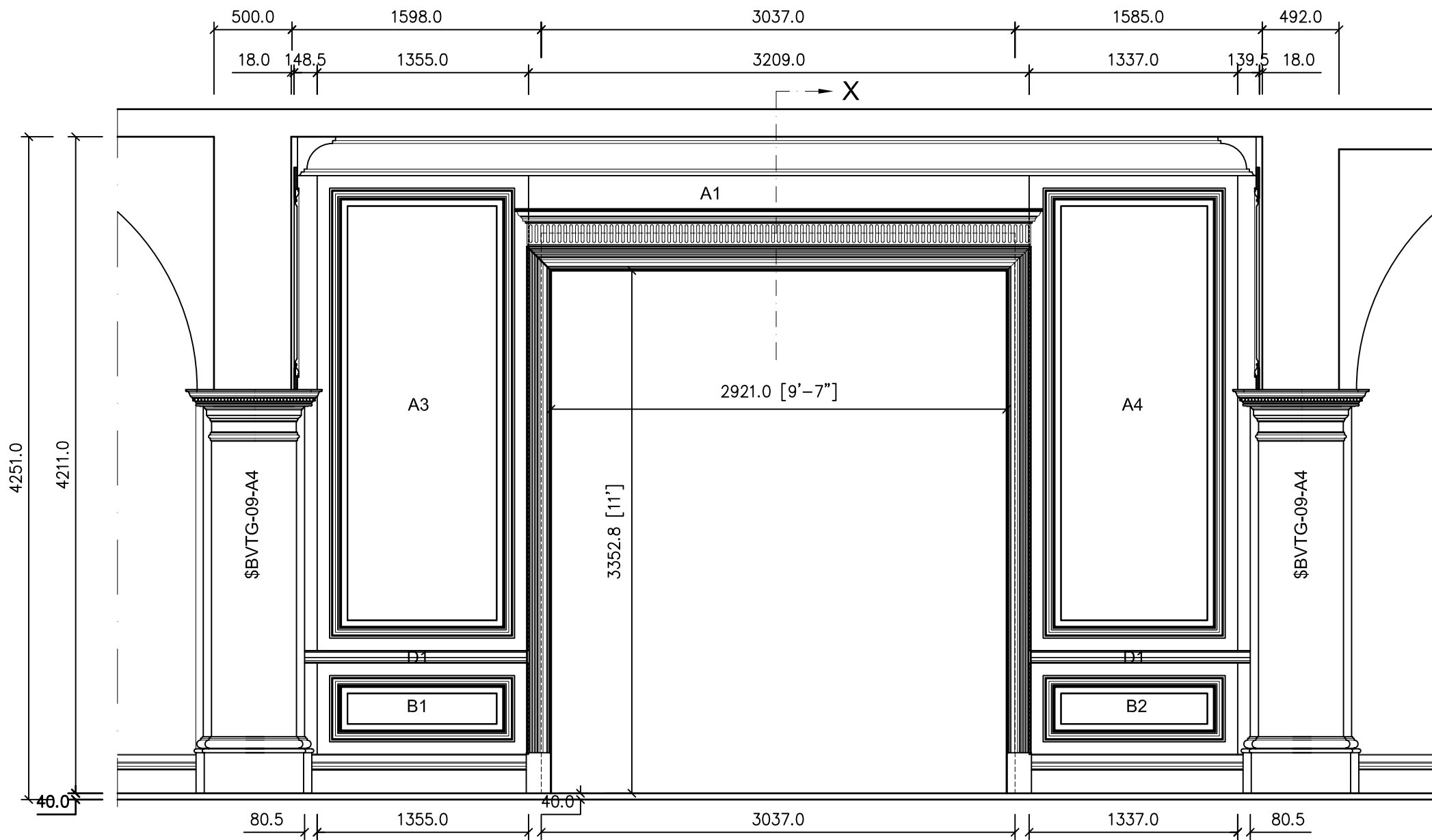
ELEVASI - A Skala 1 : 1
