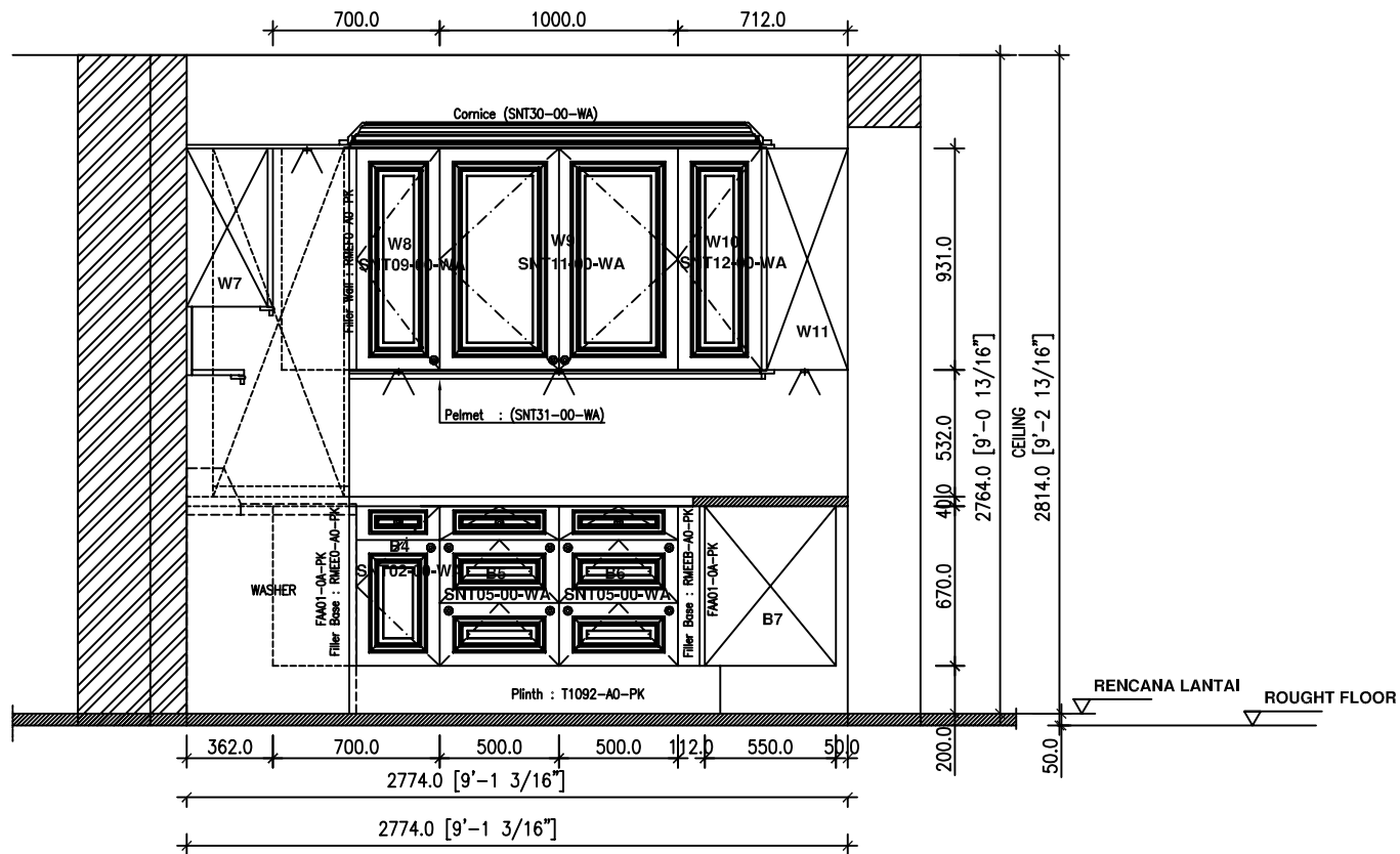
ELEVASI - C
