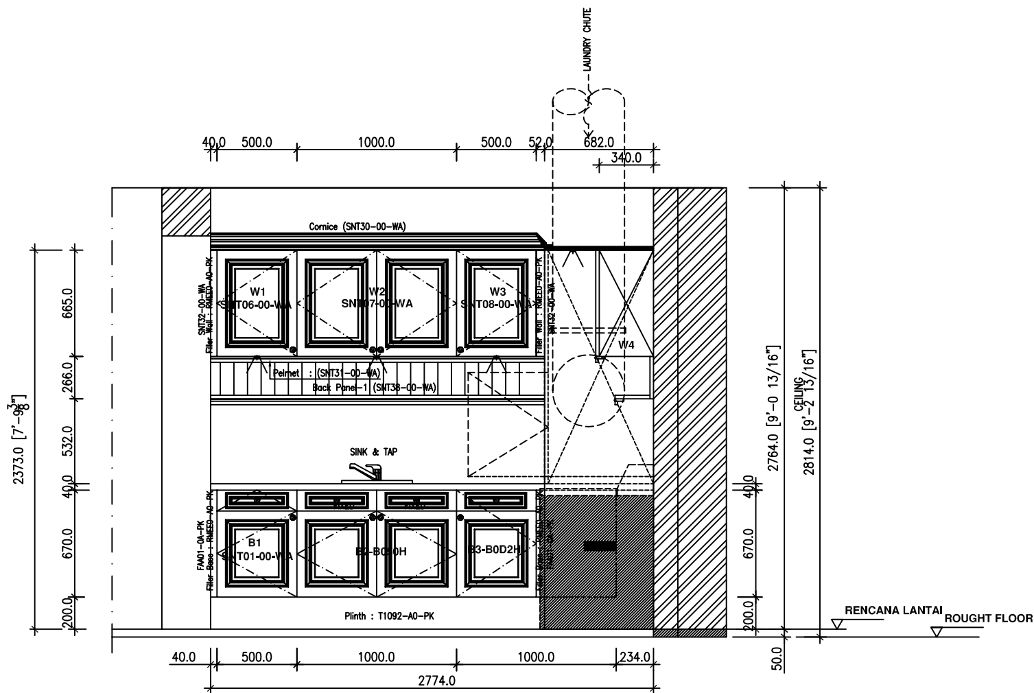
ELEVASI - A
