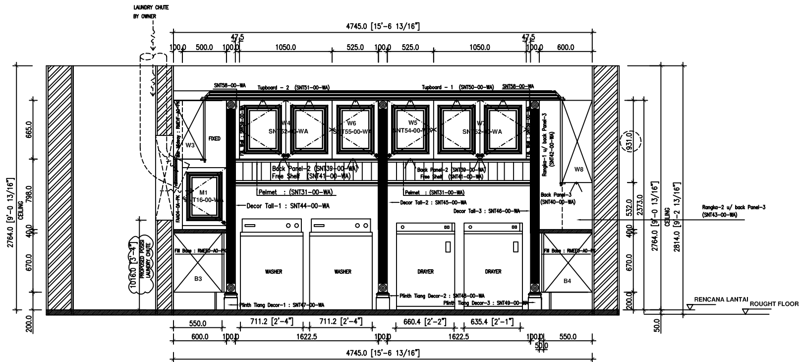
ELEVASI - B
