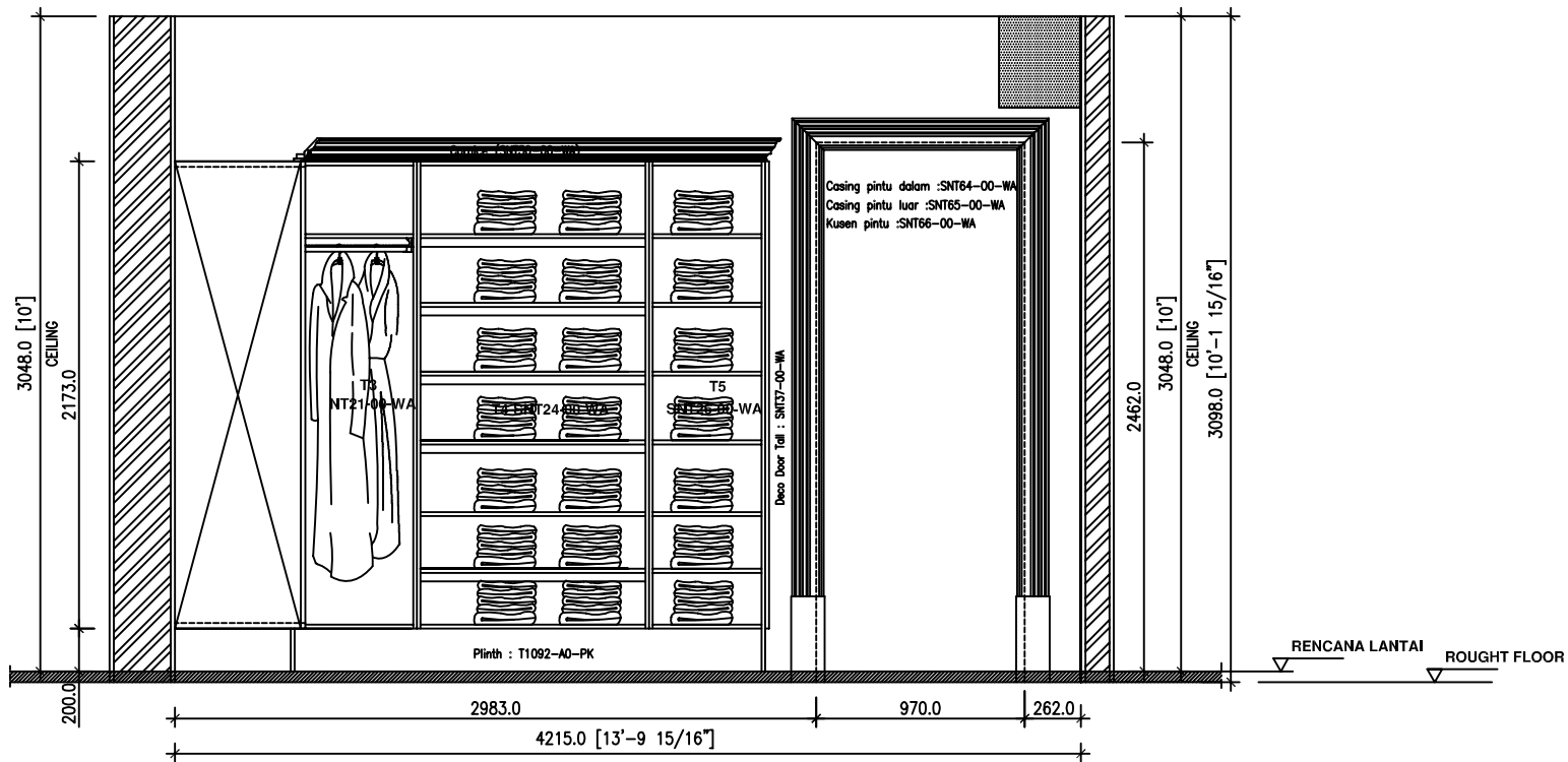
ELEVASI - F TANPA PINTU
