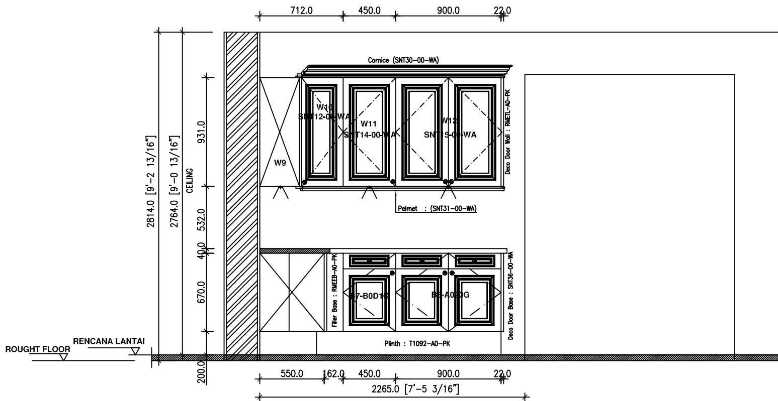
ELEVASI - D
