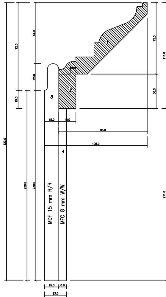
DETAIL POTONGAN A-A SKALA 1:1
