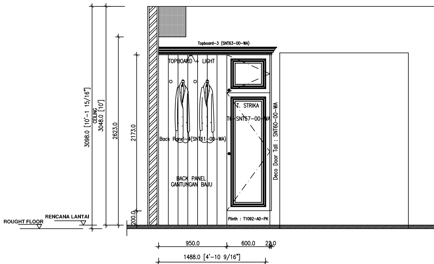
ELEVASI - G
