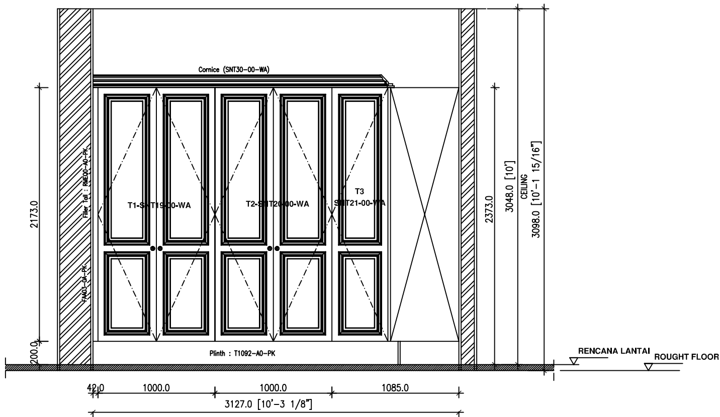
ELEVASI - E
