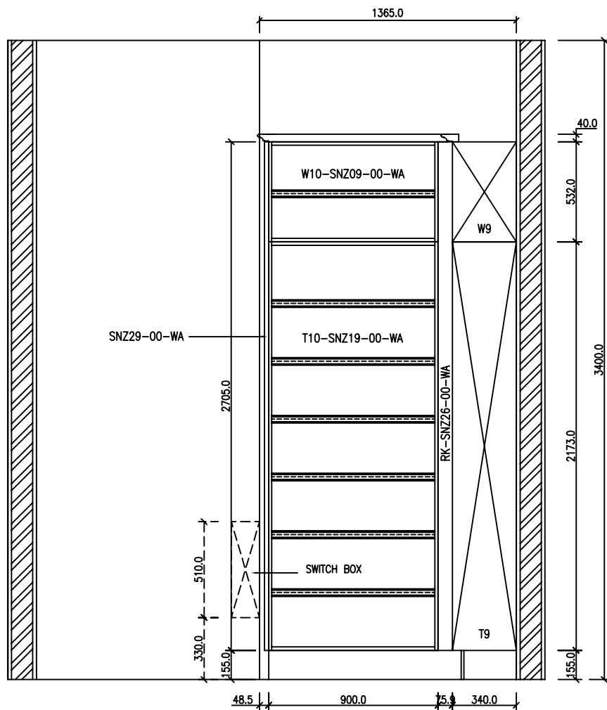
ELEVASI - E Skala 1 : 20
