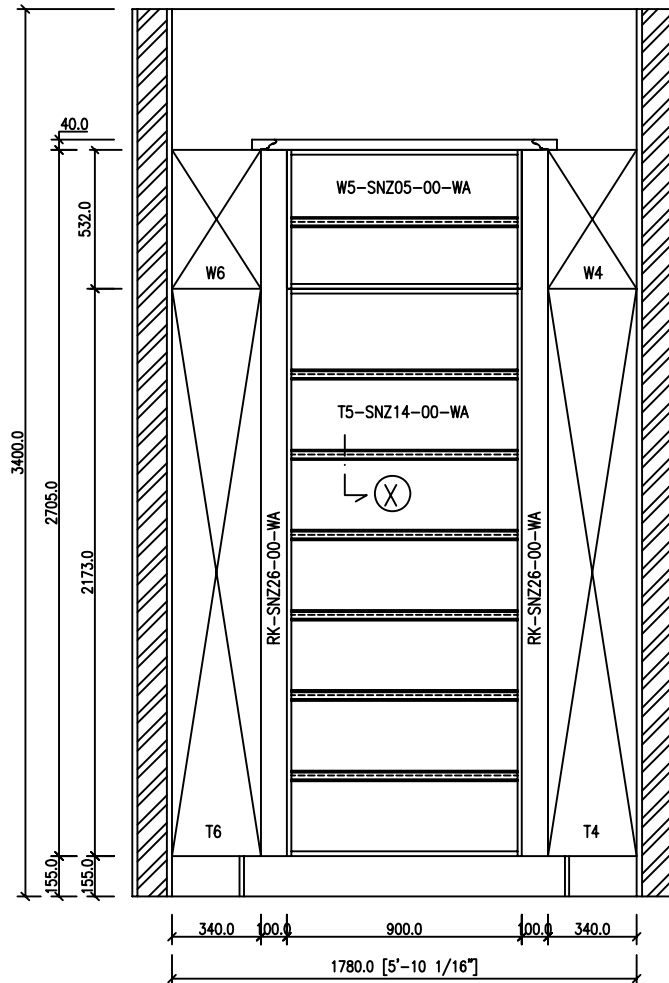
ELEVASI - C Skala 1 : 20
