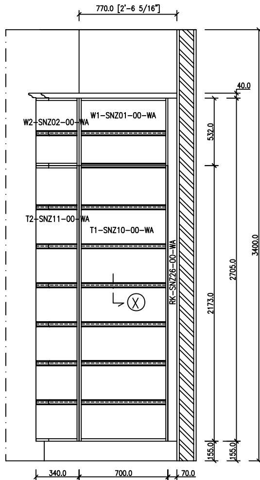
ELEVASI - A Skala 1 : 20
