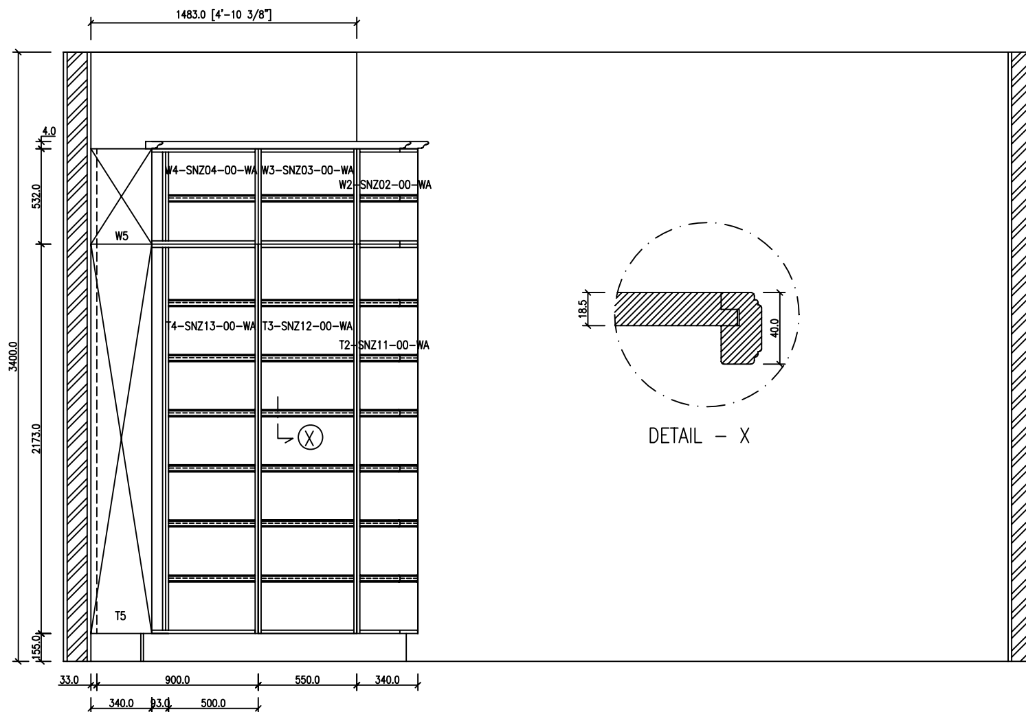
ELEVASI - B Skala 1 : 20
